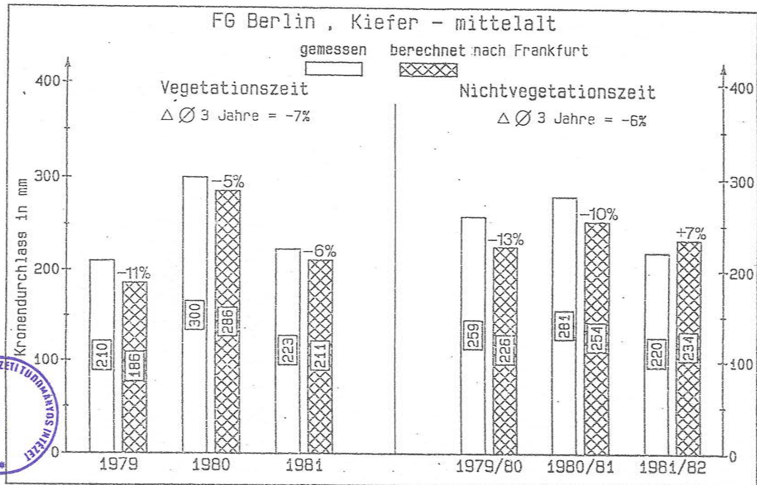
Abb. 3: Vergleich des in Berlin gemessenen Kiefer-Kronendurchlasses mit aufgrund der von Schätzbeziehungen aus Frankfurt berechneten Werte
