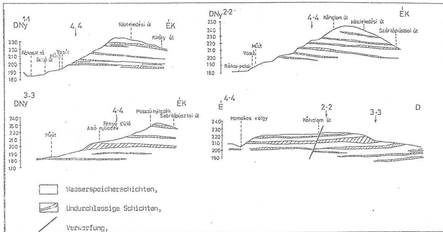
Bild 5.: AGROGEOLOGISCHE PROFILE DURCH DAS ARBORETUM VON GÖDÖLLŐ
