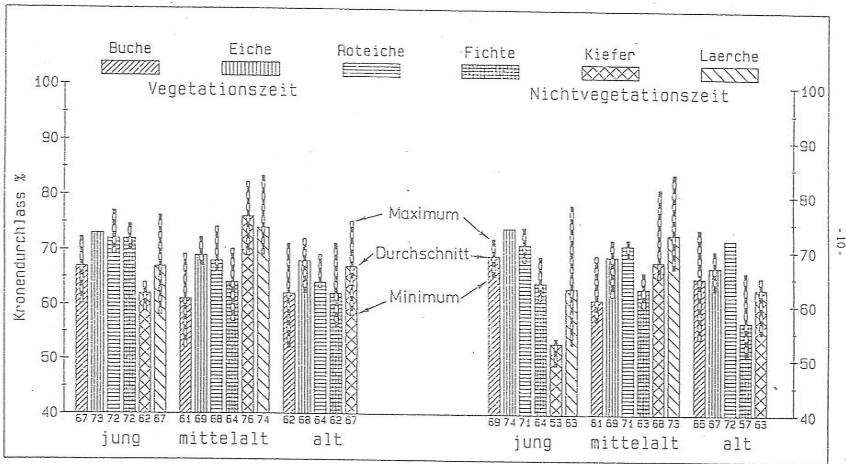
Abb. 2: Kronendurchlaßergebnisse von mehreren Beständen verschiedener Baumarten in der Vegetationszeit und in der Nichtvegetationszeit im Alter: jung, mittelalt und alt.
