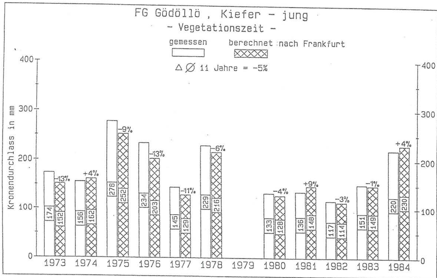
Abb. 5: Vergleich des in Gödöllő gemessenen Kiefer- (jung) Kronendurchlasses mit aufgrund der von Schätzbeziehungen aus Frankfurt berechneten Werte
