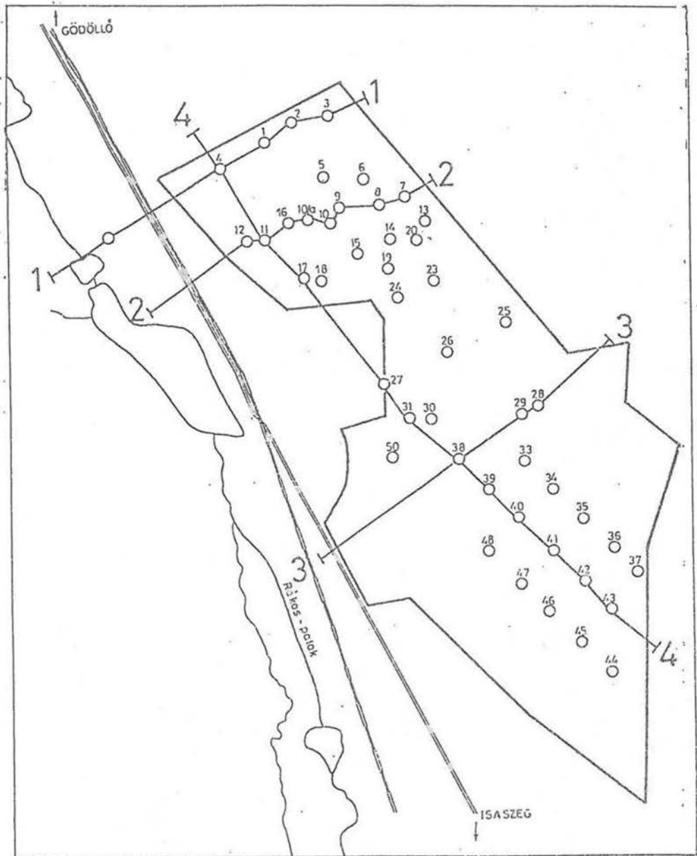
Bild 1.: DIE AGROGEOLOGISCHEN FORSCHUNGSBOHRUNGEN DES ARBORETUMS VON GÖDÖLLŐ
