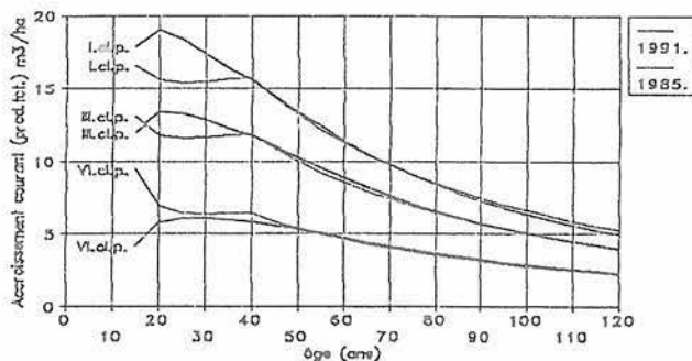
Figure 3. L'accroissement courant de la production ligneuse totale.
