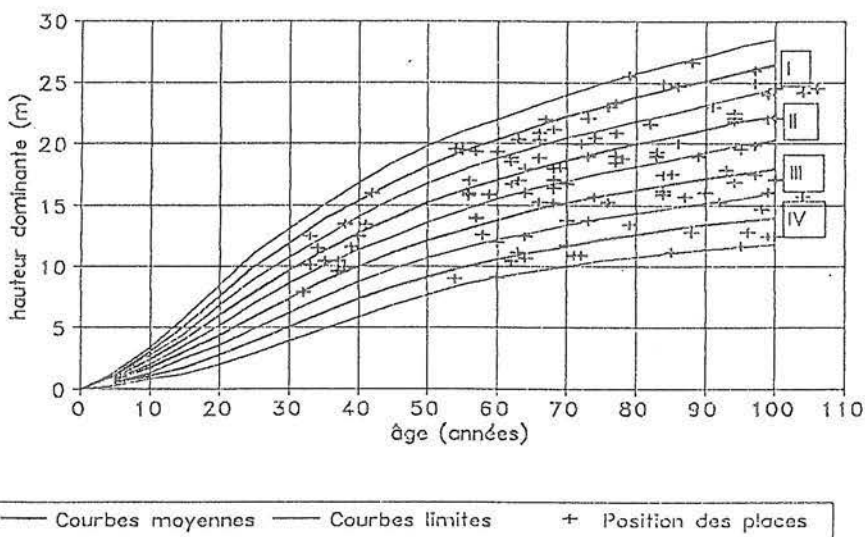
Figure 4. Classes de production construites d'après les analyses de tige par la méthode graphique
