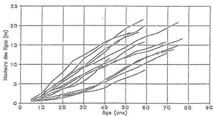
Figure 2. Données des analyses des tiges. L'allure de la croissance en hauteur.
