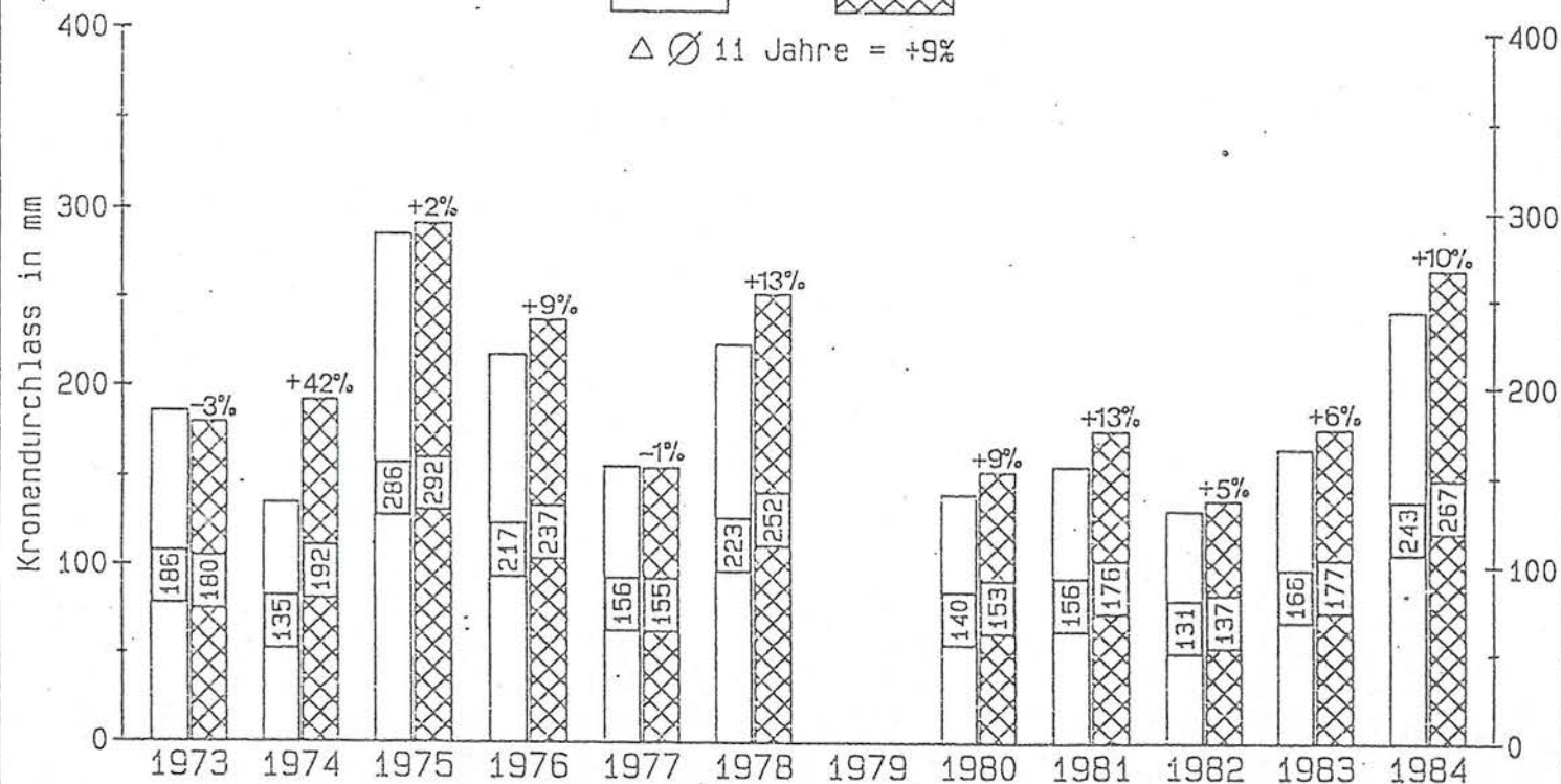
Abb. 4: Vergleich des in Gödöllő gemessenen Kiefer- (mittelalt) Kronendurchlasses mit aufgrund der von Schätzbeziehungen aus Frankfurt berechneten Werte
