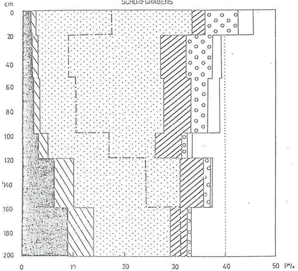
Bild 4.: DIFFERENZIERTE PORENVERTETLUNG DER SEDIMENTE DES SCHURFGRABENS
