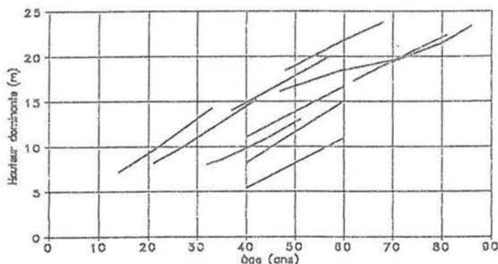
Figure 1. L'allure de croissance de la hauteur dominante
