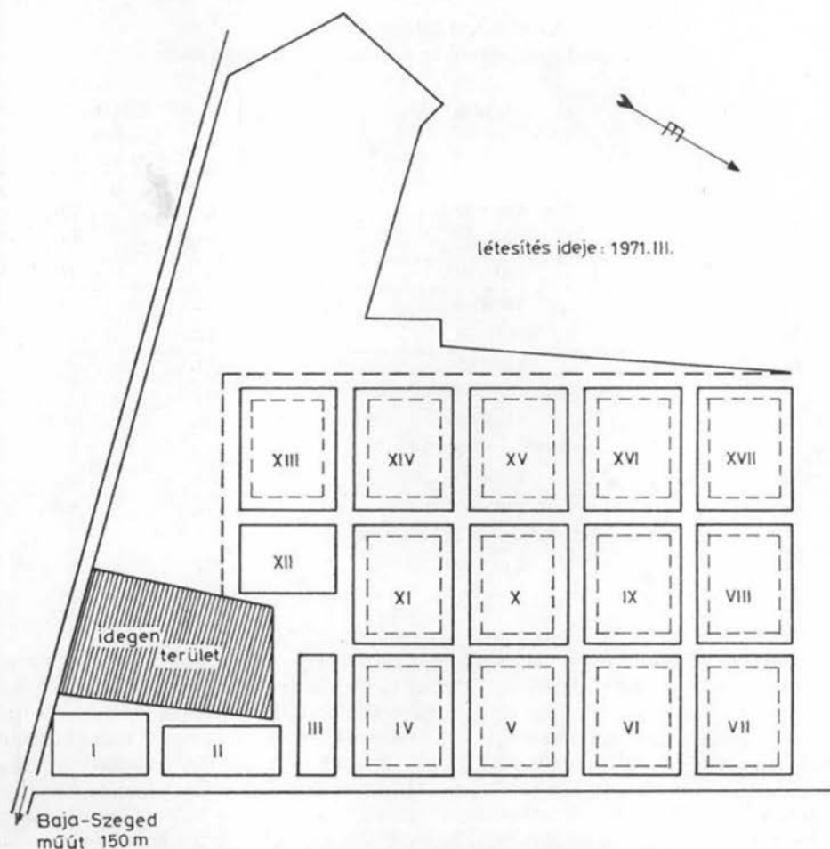
1. ábra. Ásotthalom 68 H/1978 erdeifenyő-ültetés hálózati kísérlete Figure 1. Design of a long-term Scots pine spacing experiment, Ásotthalom, 68 H
