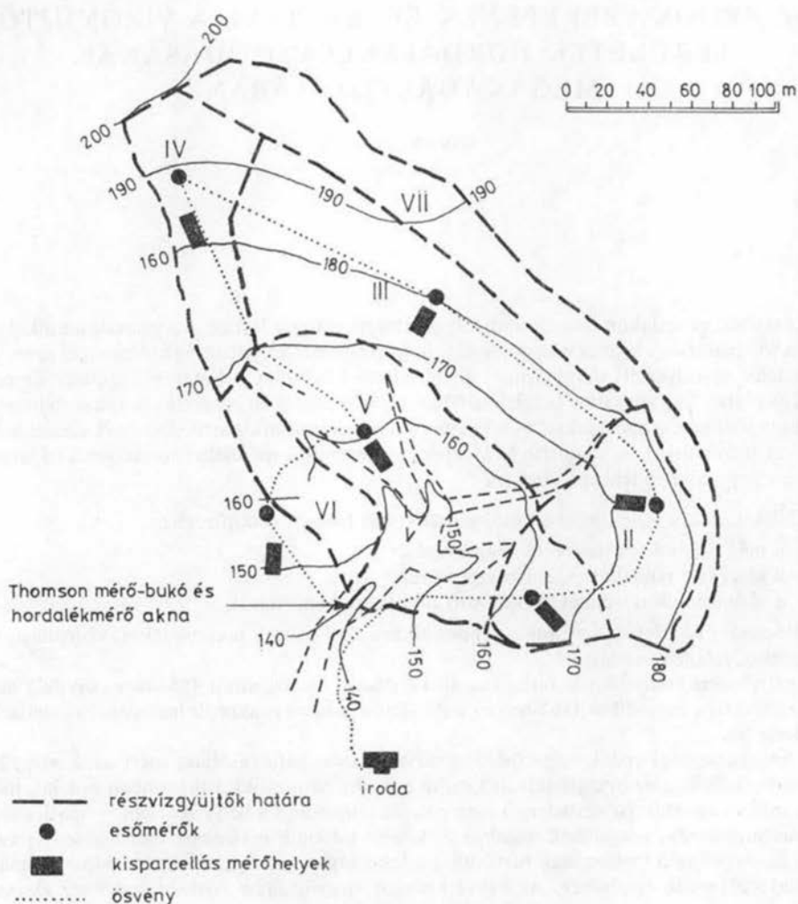
1. ábra. ERTI eróziómérő állomás Kisnána
