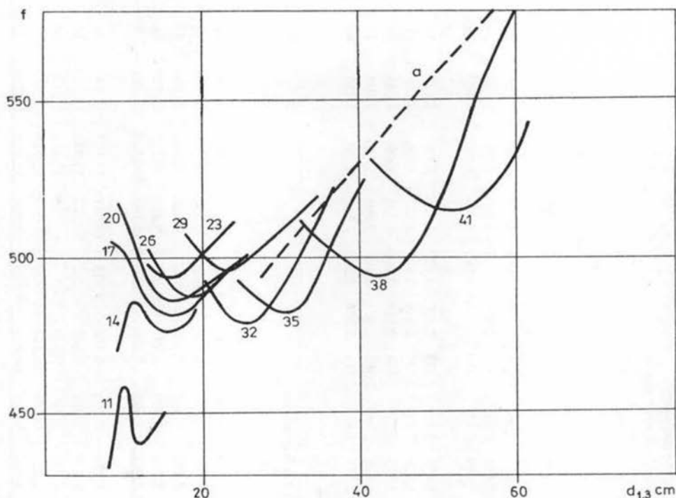
3. ábra. Az új kiegyenlített vastagfa-alakszám-görbék alsó szakasza magassági csoportok szerint az átmérő függvényében
