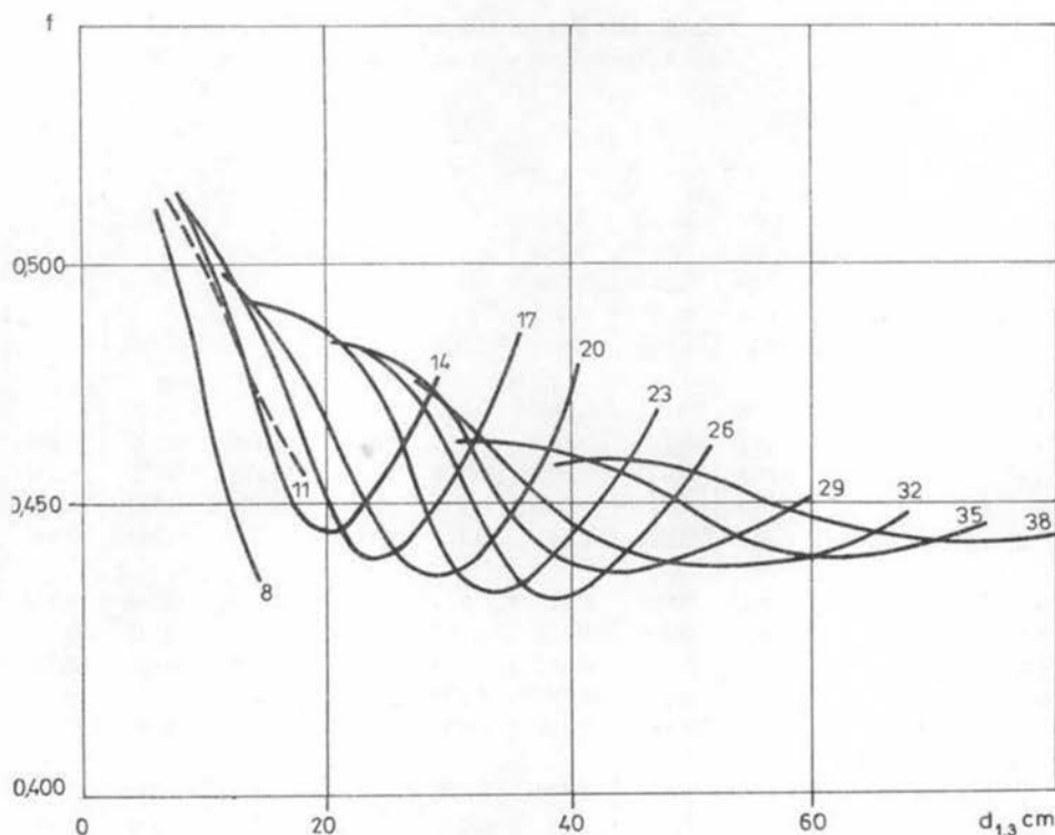
2. ábra. Új törzsfaalakszámok a magassági csoportok szerint az átmérő függvényében
