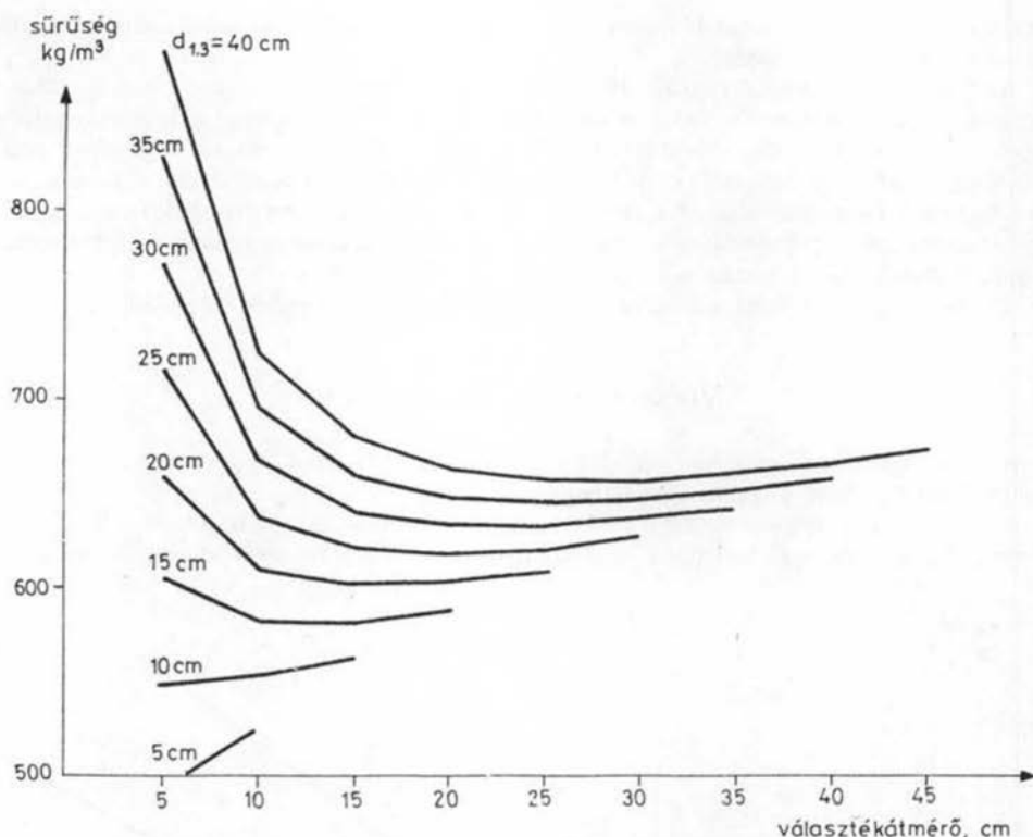
2. ábra. Akác sűrűsége átlalóval kéregben mért térfogatra vonatkoztatva a mellmagassági átmérő és a választékátmérő függvényében
