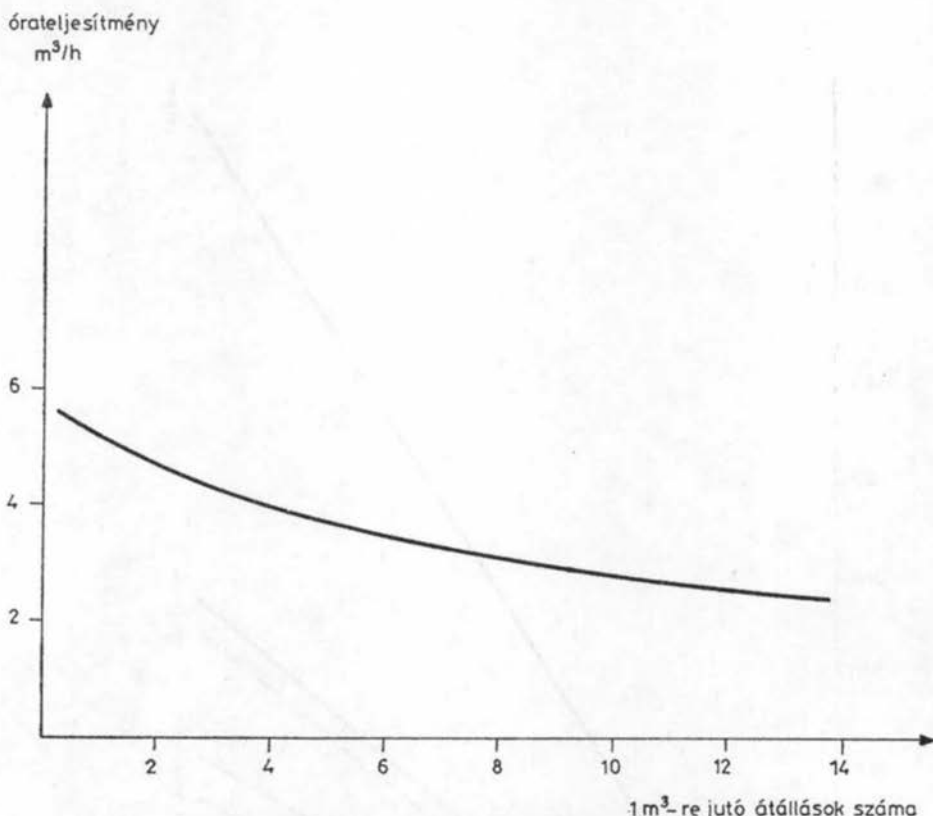
2. ábra. Az aprítékkészítés teljesítménye az átállásgyakoriság függvényében
