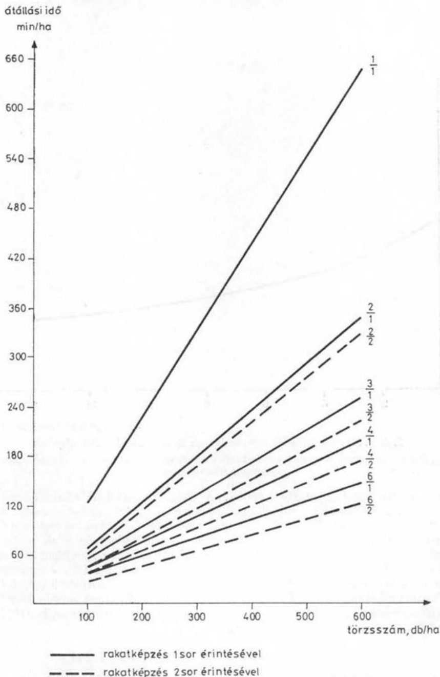
1. ábra. A hektáronkénti átállásiidő-szükséglet a törzsszám függvényében különböző koncentrációs mód esetében
